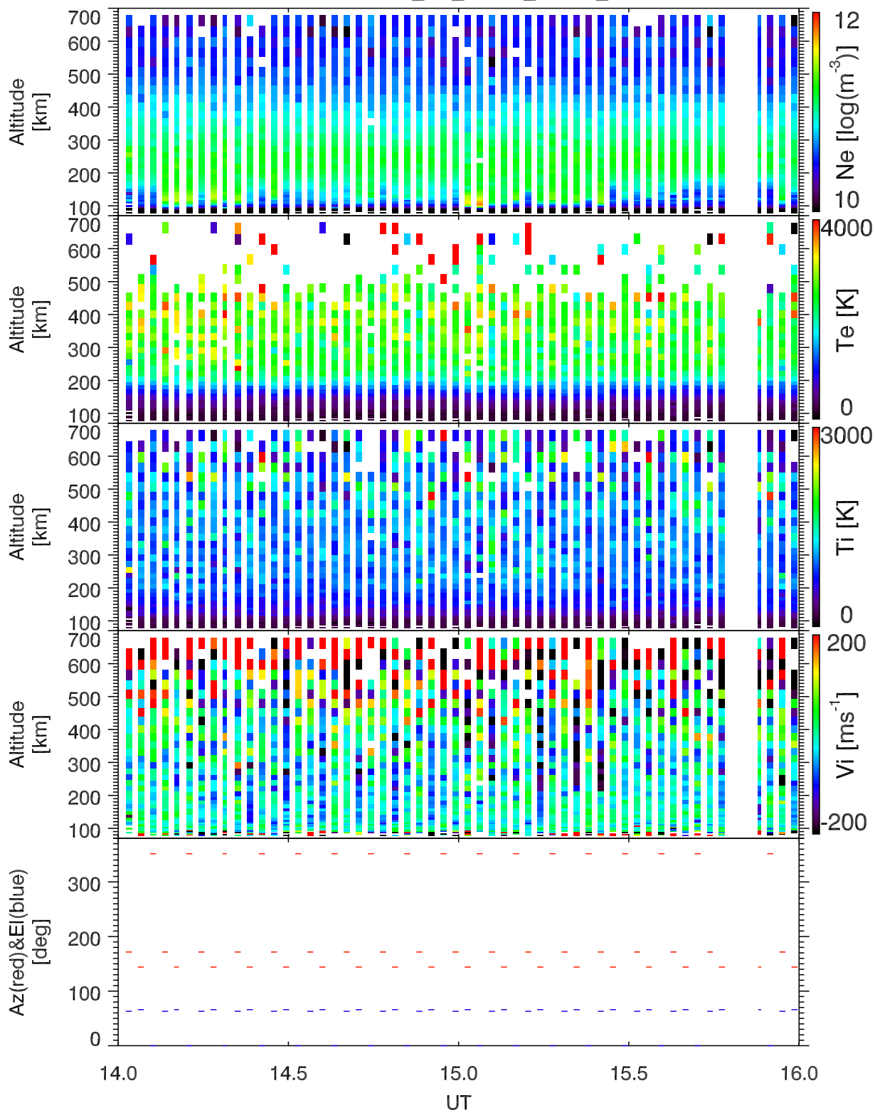
EISCAT 2005-09-05_14_16UT_steffe_ant@32m.
