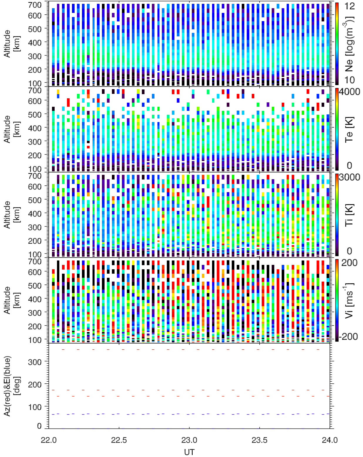
EISCAT 2005-09-05_22_24UT_steffe_ant@32m.
