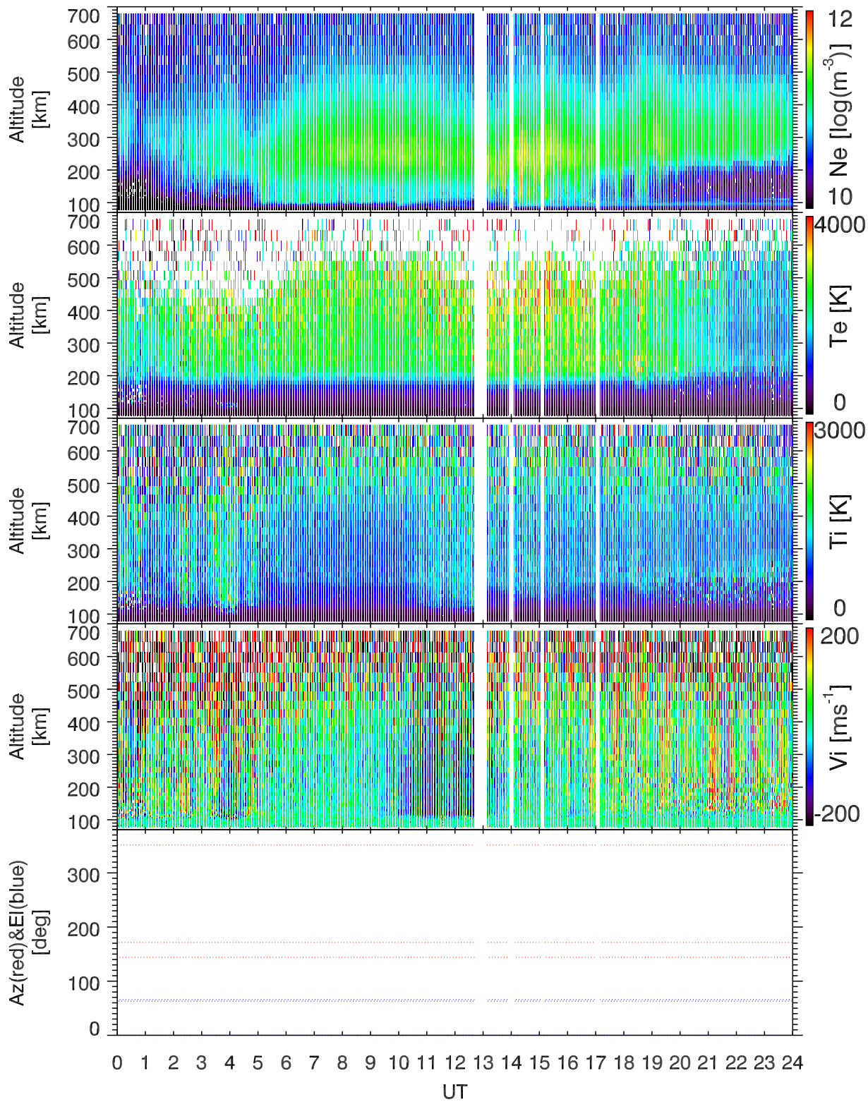
EISCAT 2005-09-09_00_24UT_steffe_ant@32m.
