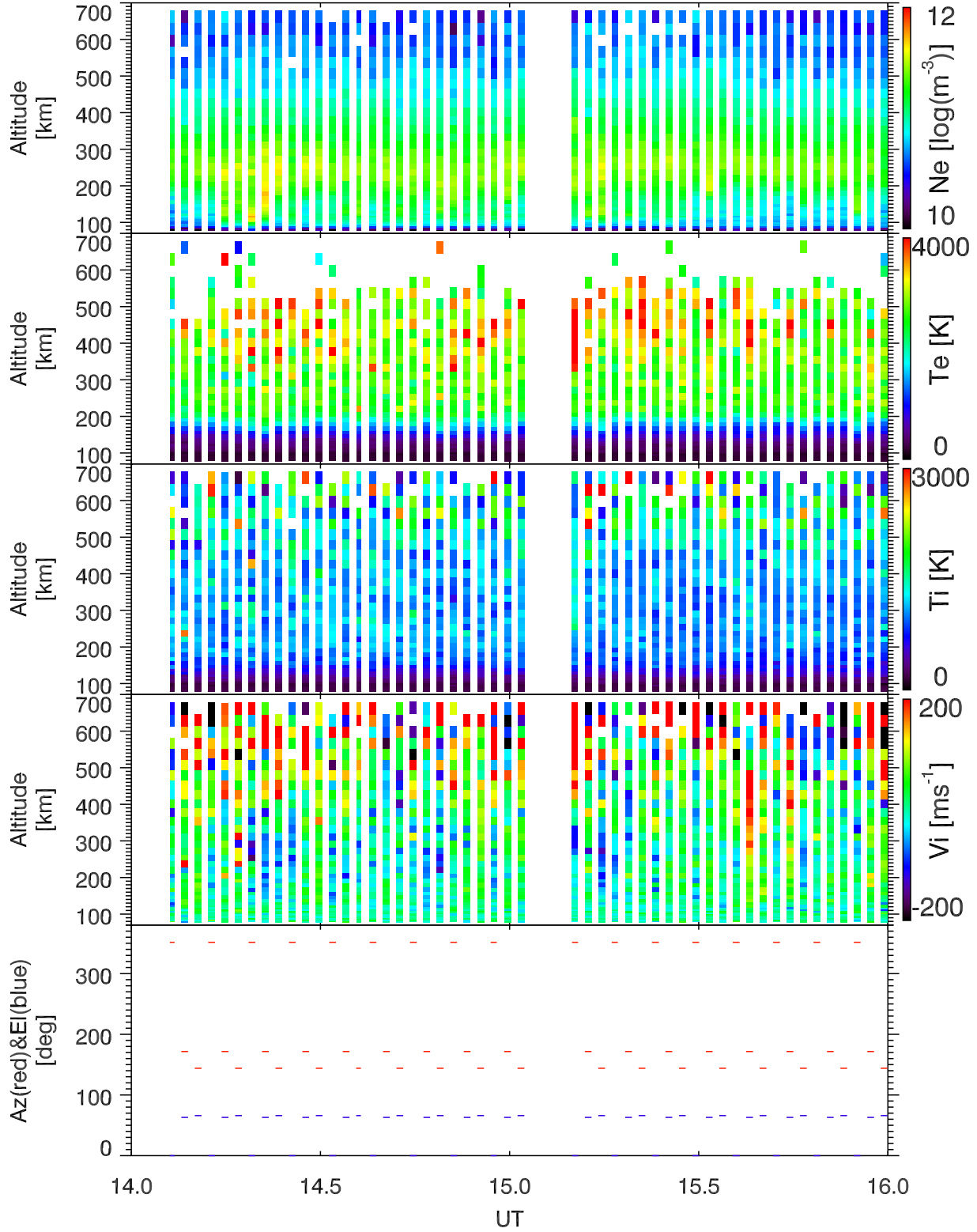
EISCAT 2005-09-09_14_16UT_steffe_ant@32m.
