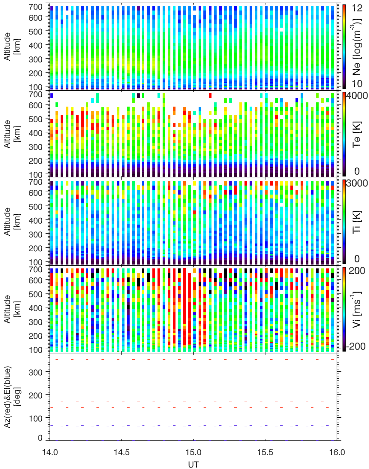
EISCAT 2005-09-10_14_16UT_steffe_ant@32m.
