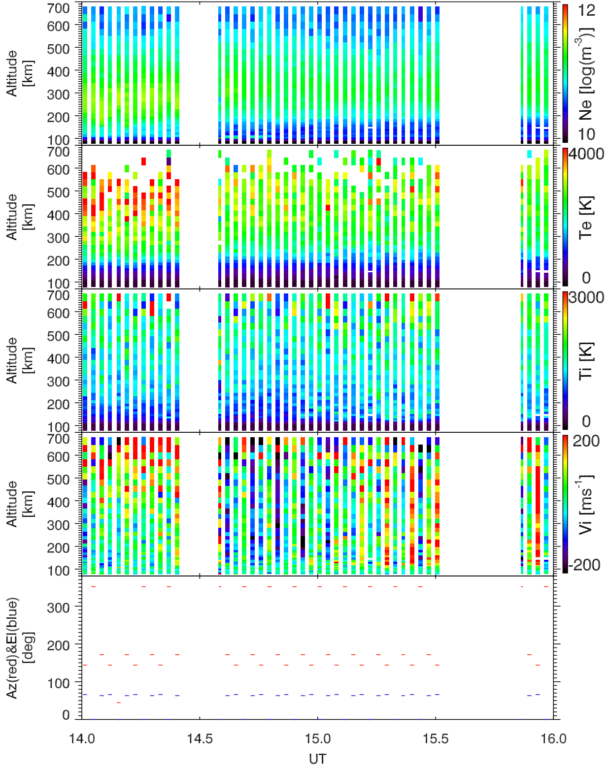
EISCAT 2005-09-12_14_16UT_steffe_ant@32m.
