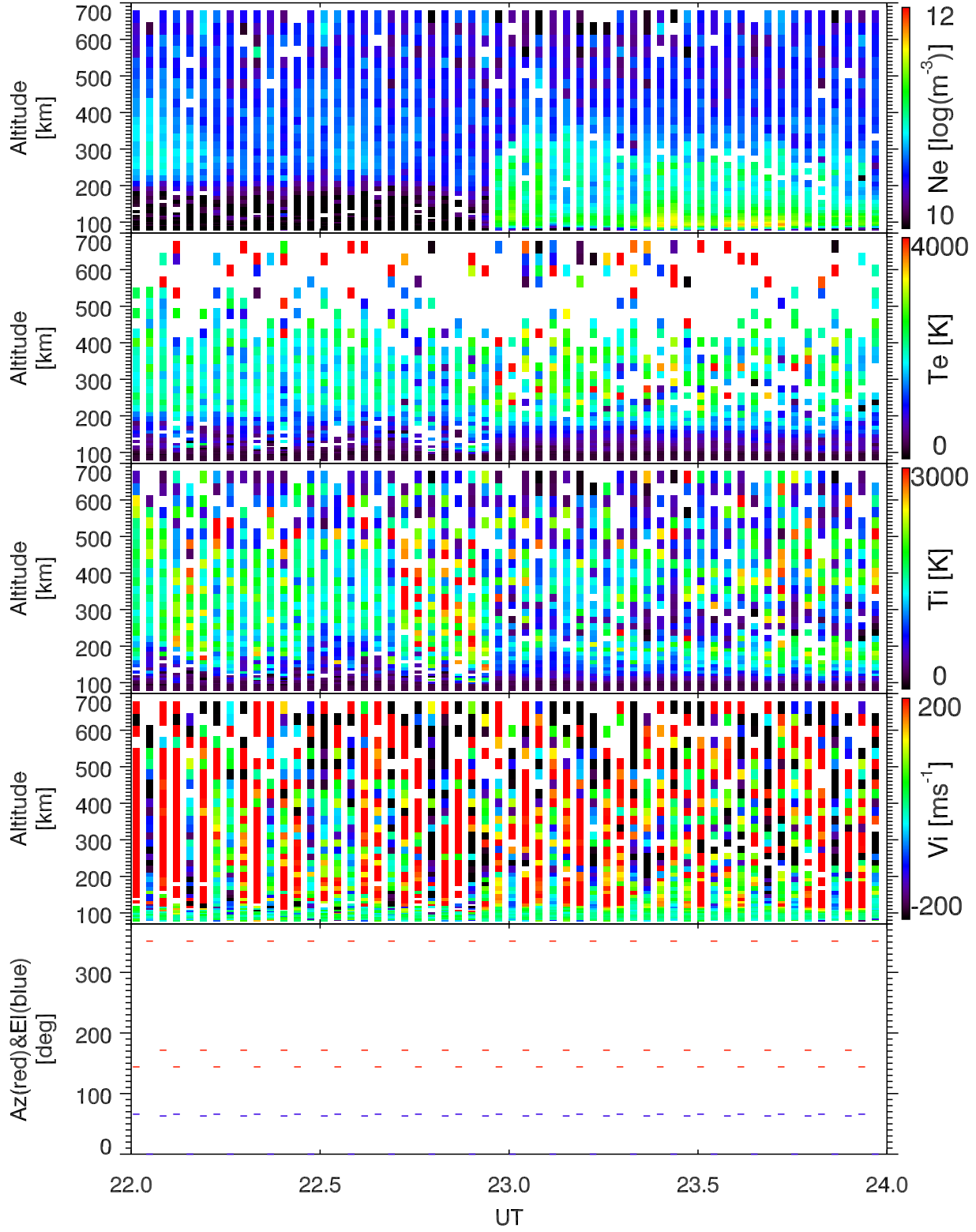
EISCAT 2005-09-12_22_24UT_steffe_ant@32m.
