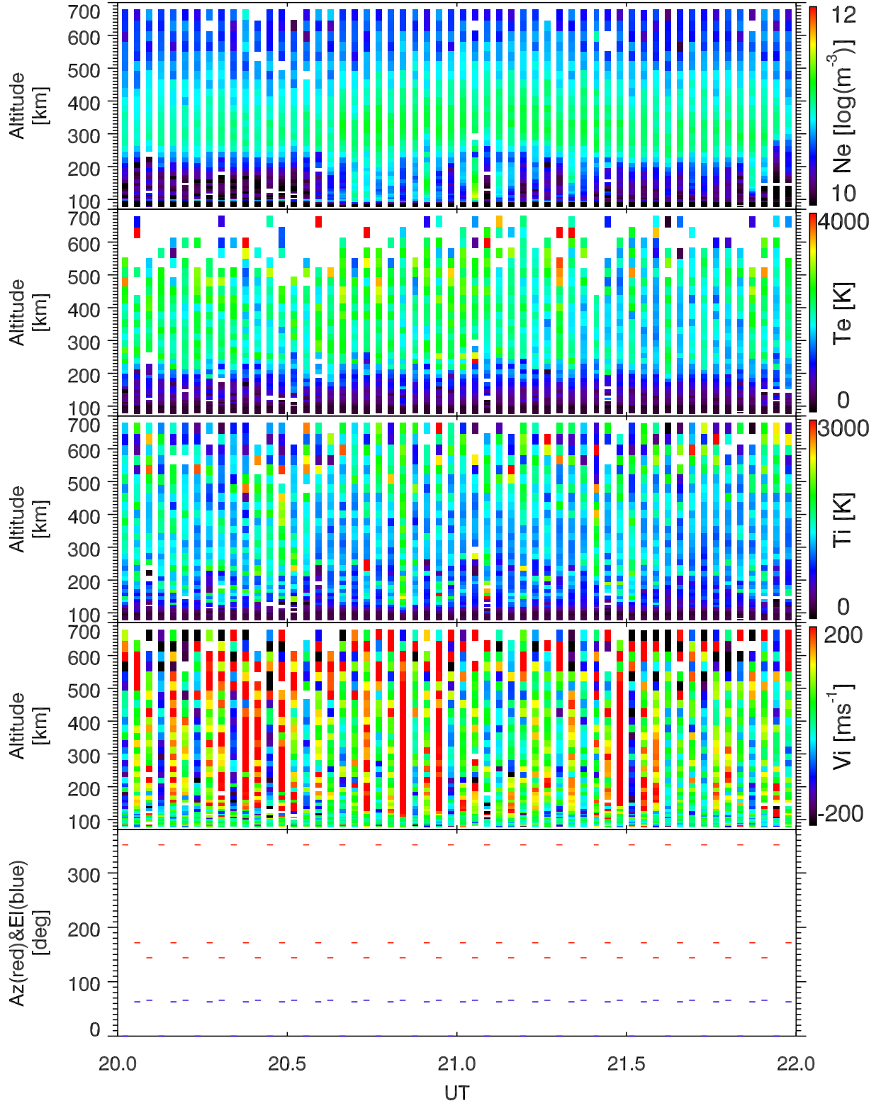
EISCAT 2005-09-13_20_22UT_steffe_ant@32m.
