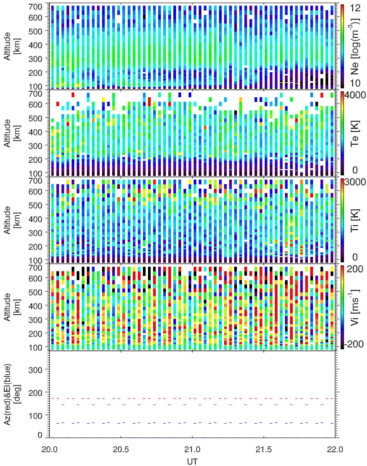
EISCAT 2005-09-14_20_22UT_steffe_ant@32m.
