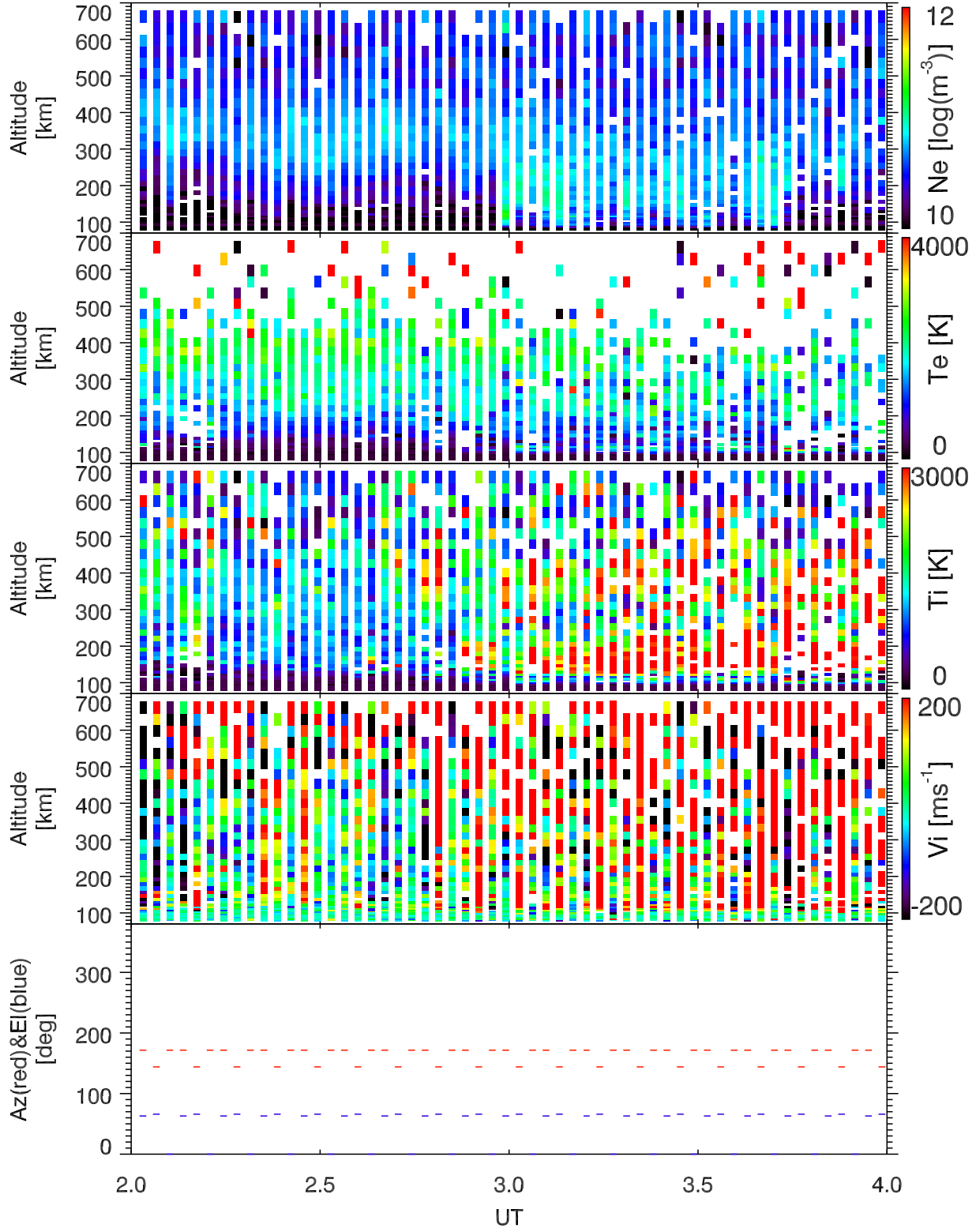
EISCAT 2005-09-16_02_04UT_steffe_ant@32m.
