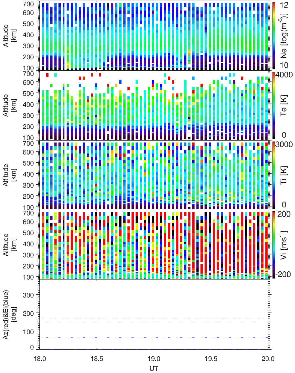
EISCAT 2005-09-16_18_20UT_steffe_ant@32m.
