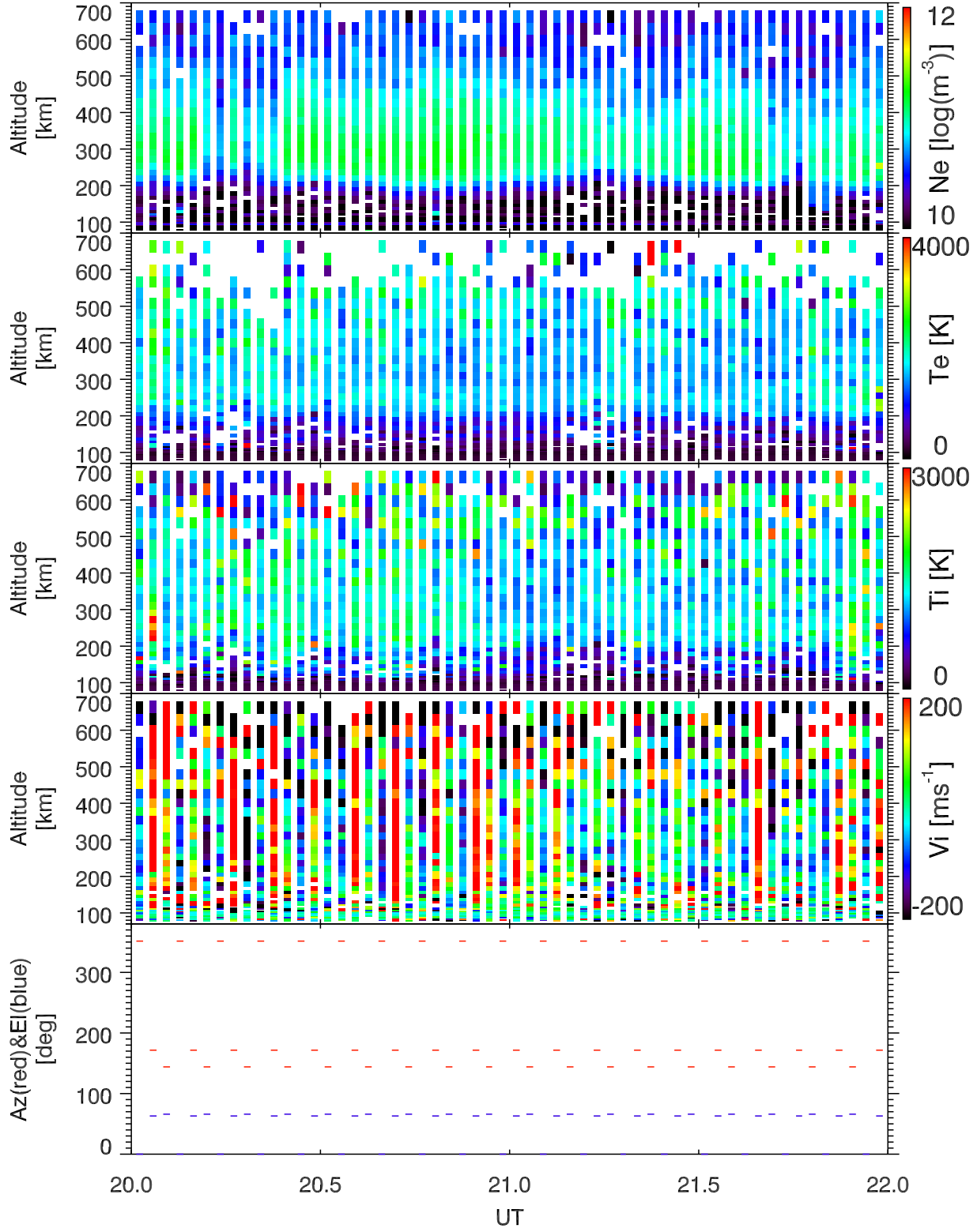
EISCAT 2005-09-17_20_22UT_steffe_ant@32m.
