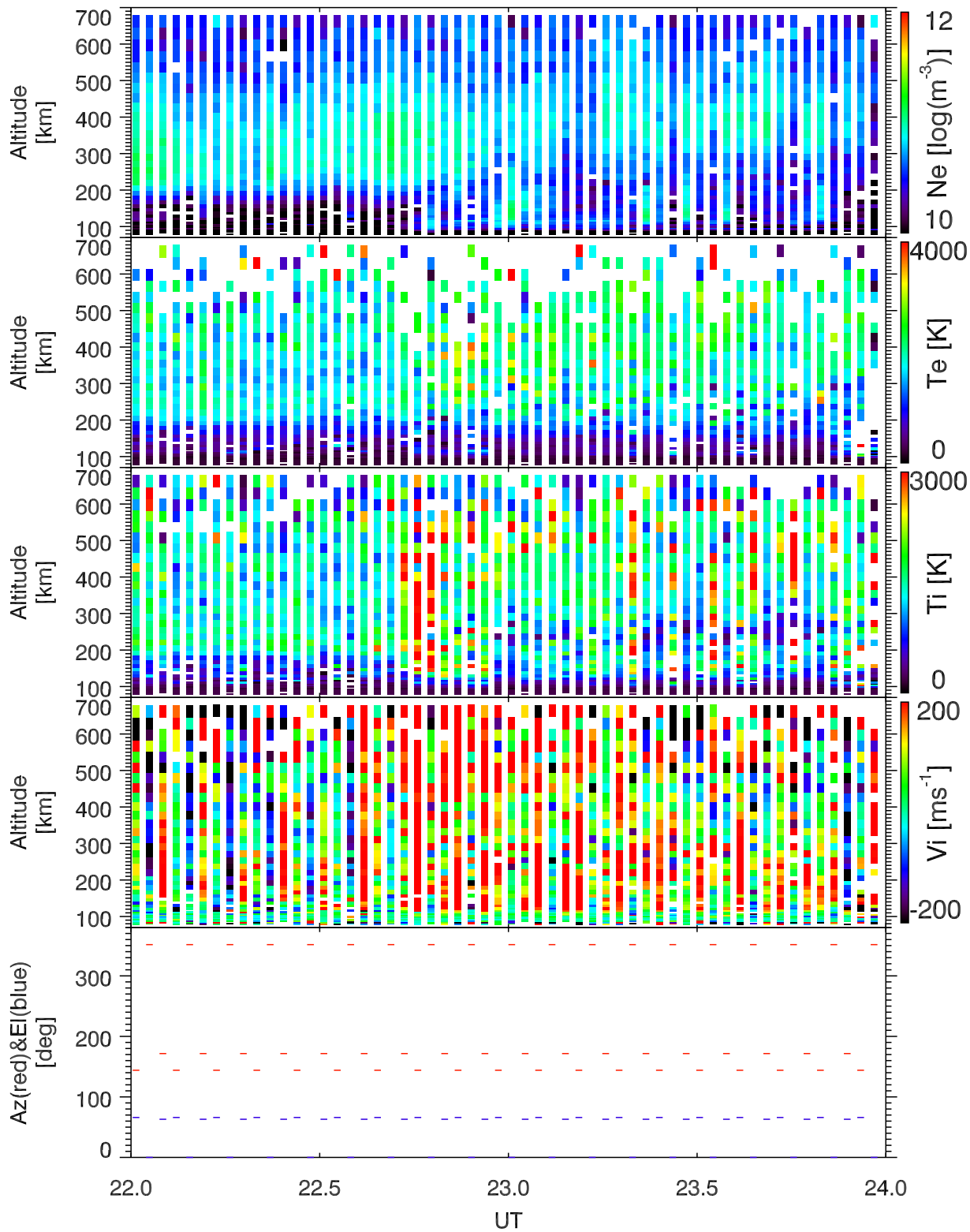
EISCAT 2005-09-17_22_24UT_steffe_ant@32m.
