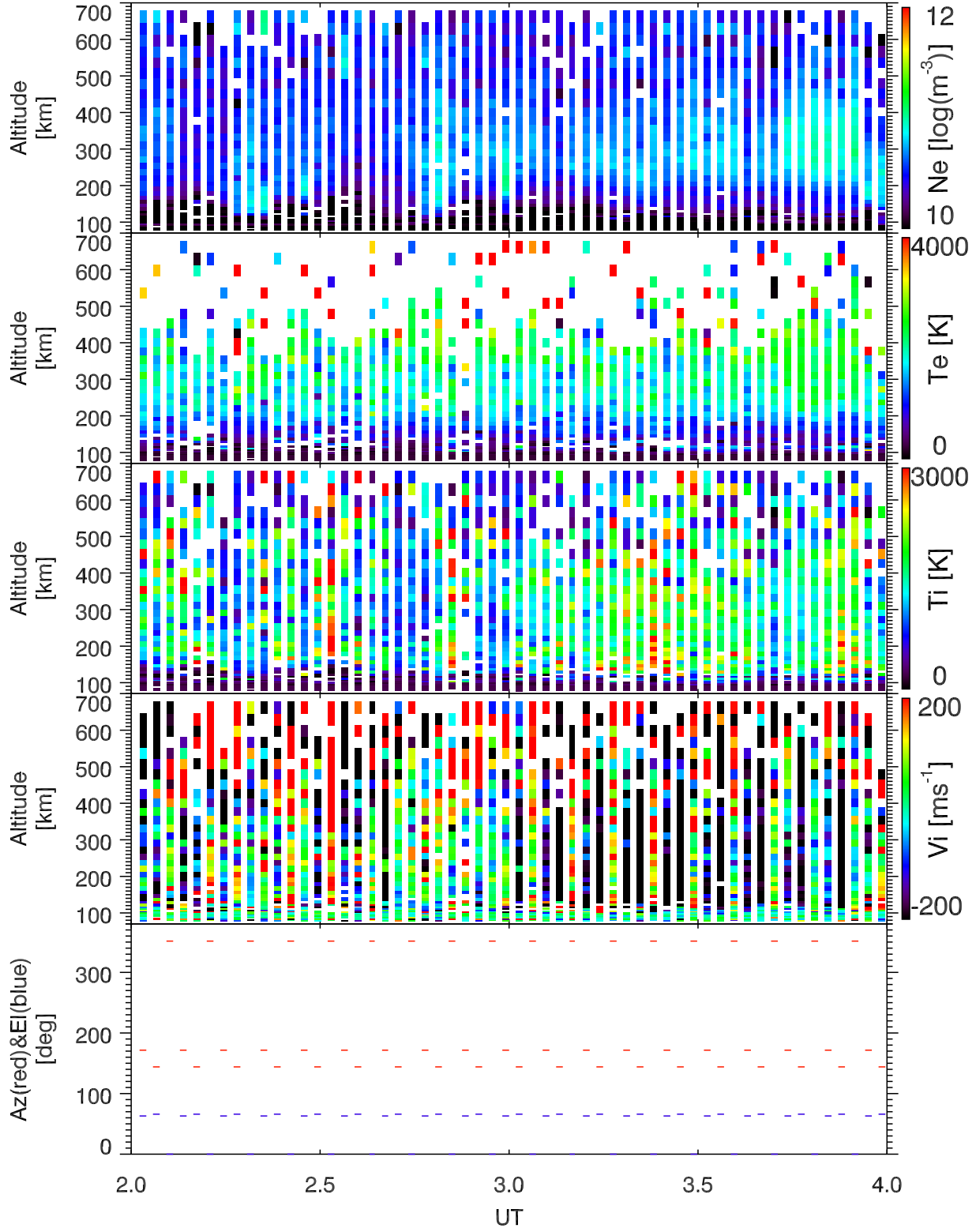
EISCAT 2005-09-18_02_04UT_steffe_ant@32m.
