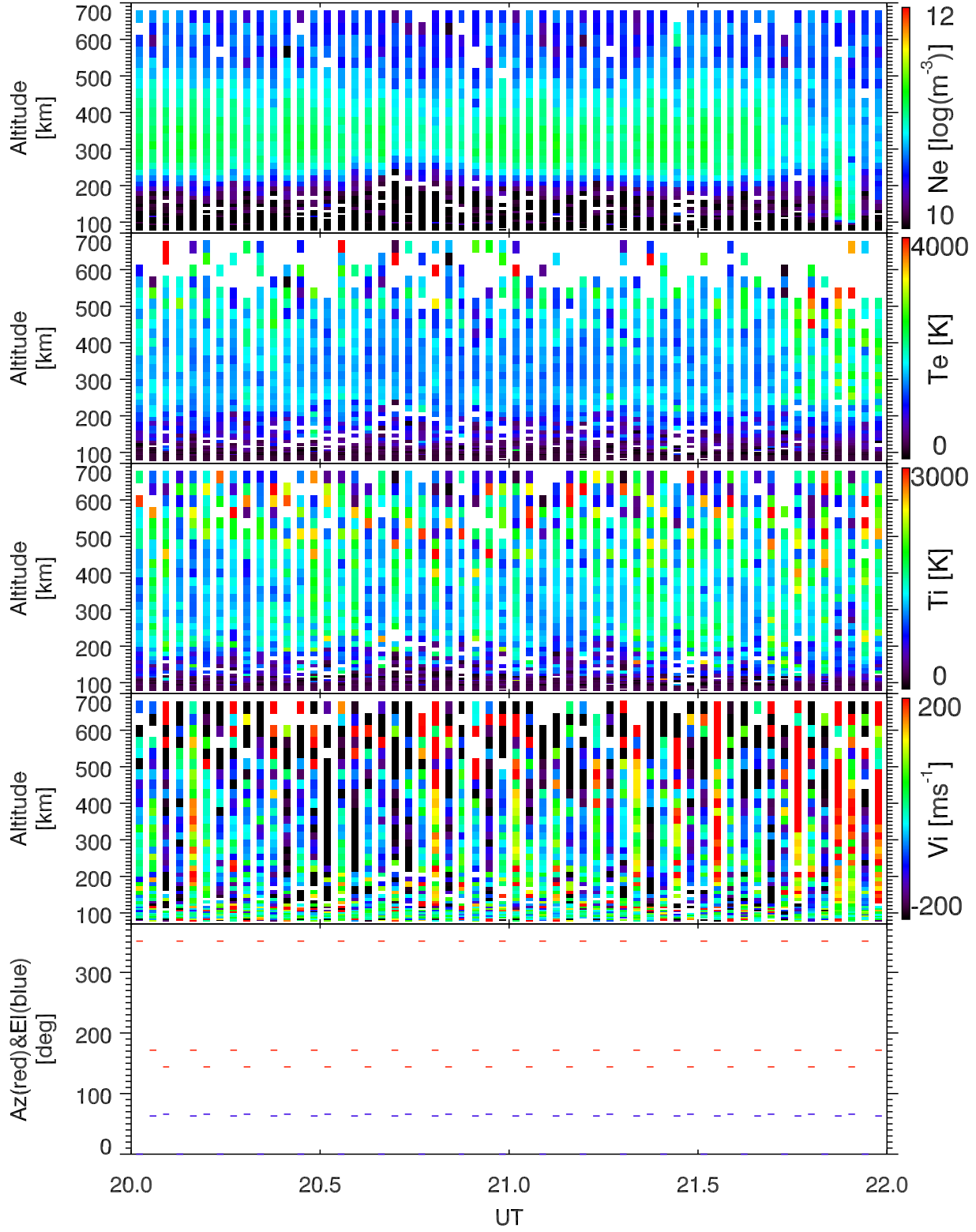
EISCAT 2005-09-18_20_22UT_steffe_ant@32m.
