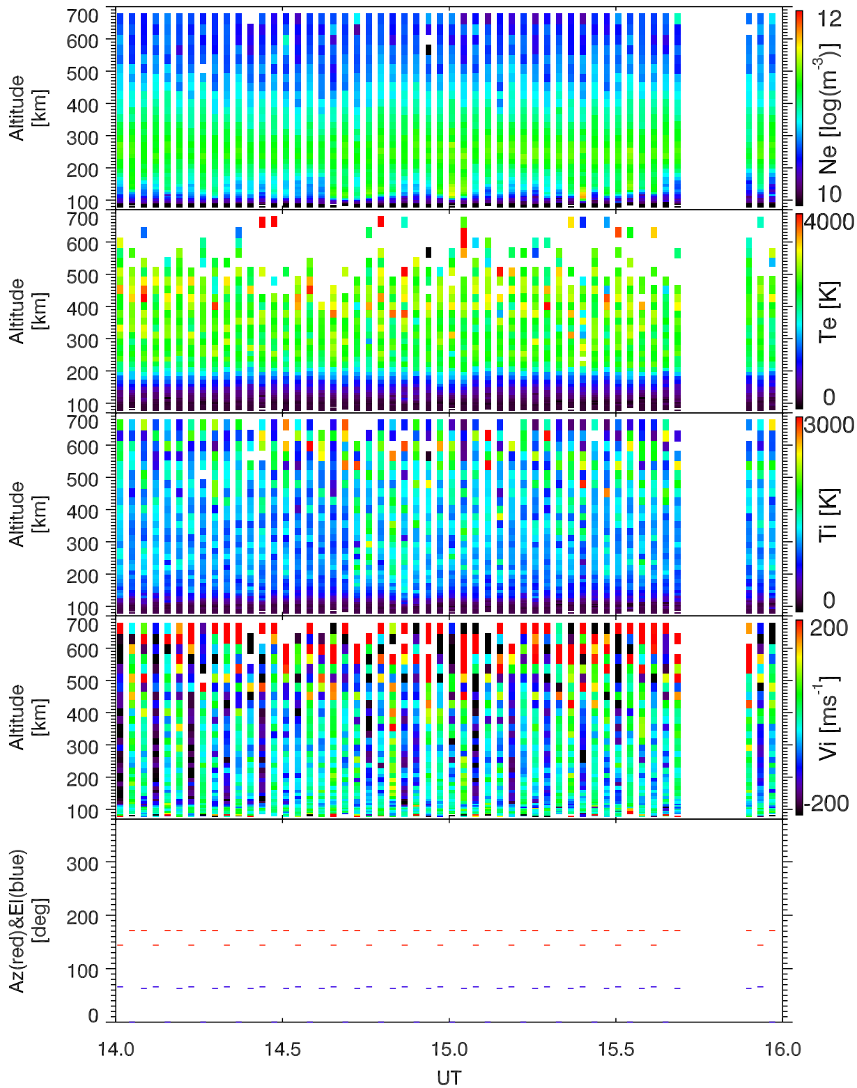
EISCAT 2005-09-19_14_16UT_steffe_ant@32m.
