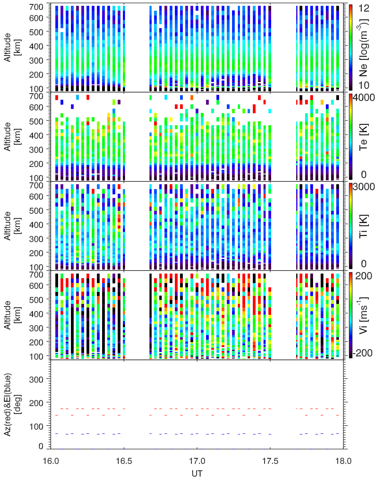
EISCAT 2005-09-21_16_18UT_steffe_ant@32m.
