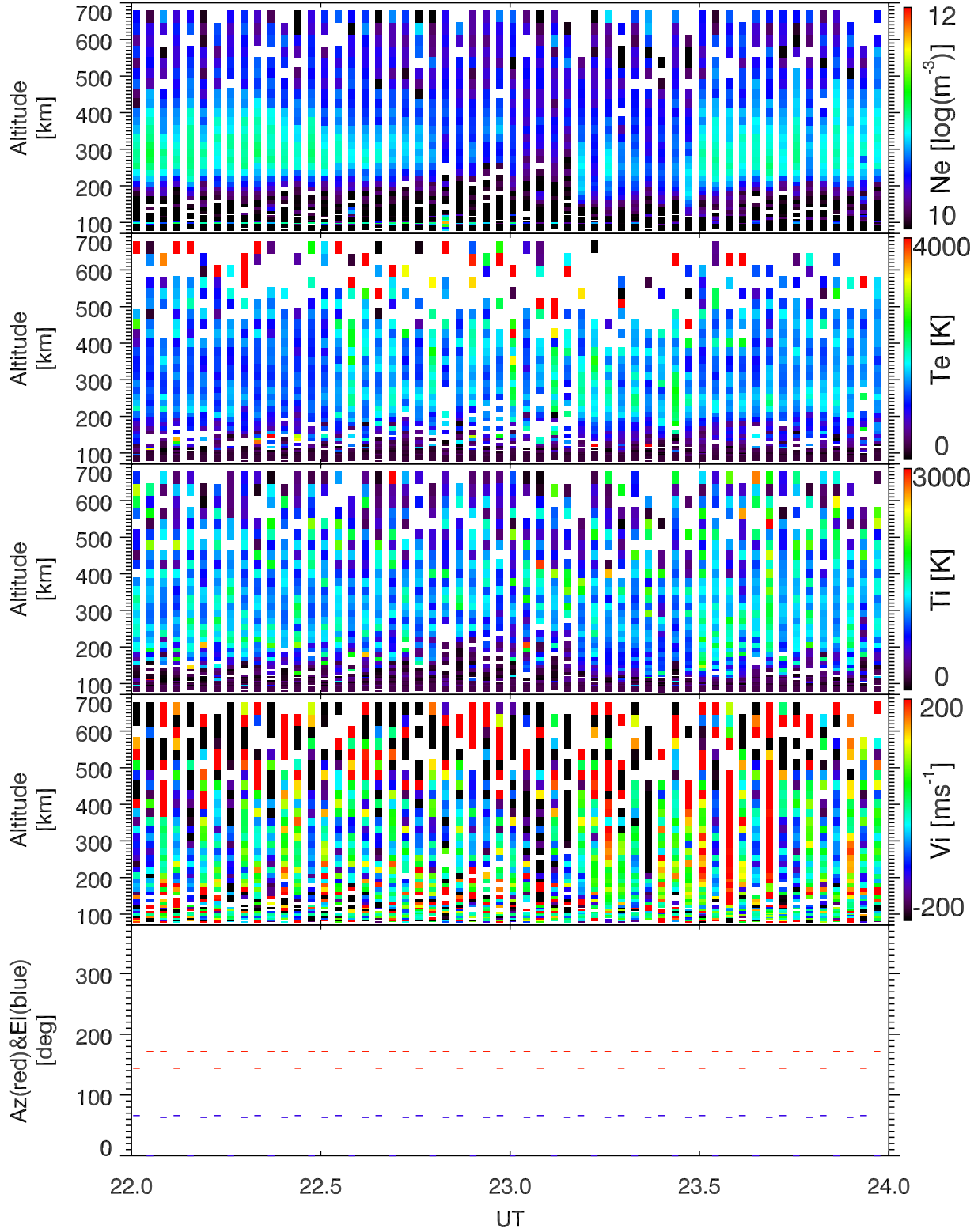
EISCAT 2005-09-21_22_24UT_steffe_ant@32m.
