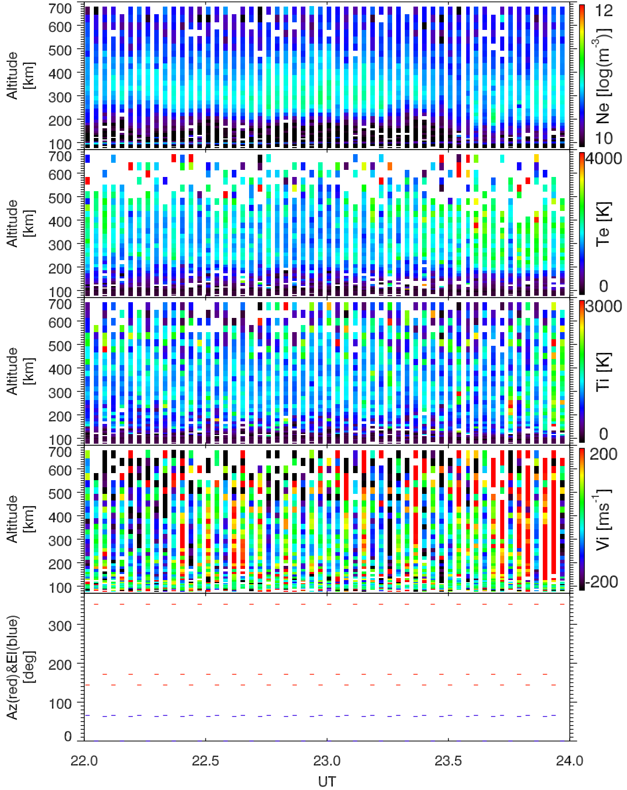
EISCAT 2005-09-22_22_24UT_steffe_ant@32m.
