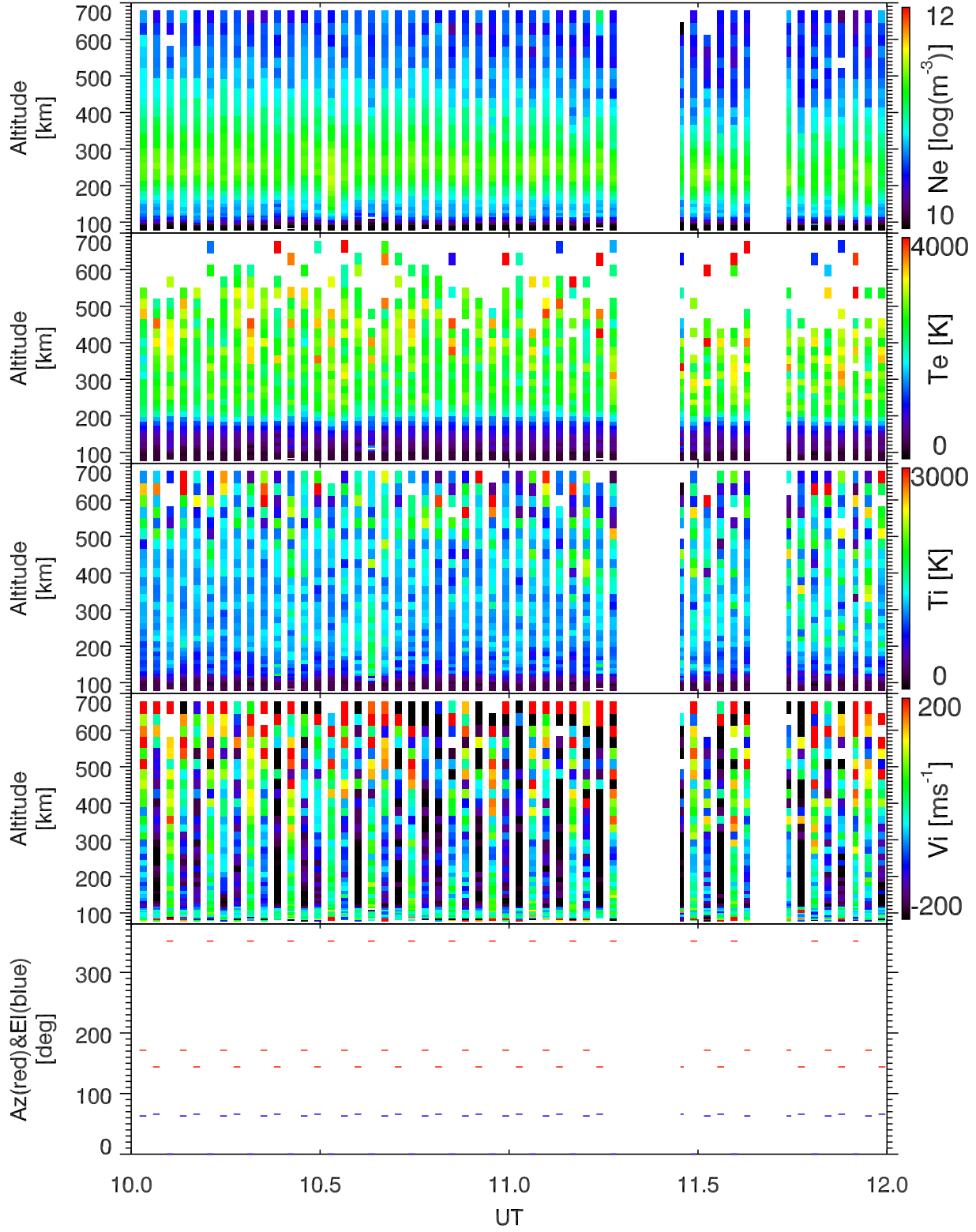
EISCAT 2005-09-23_10_12UT_steffe_ant@32m.
