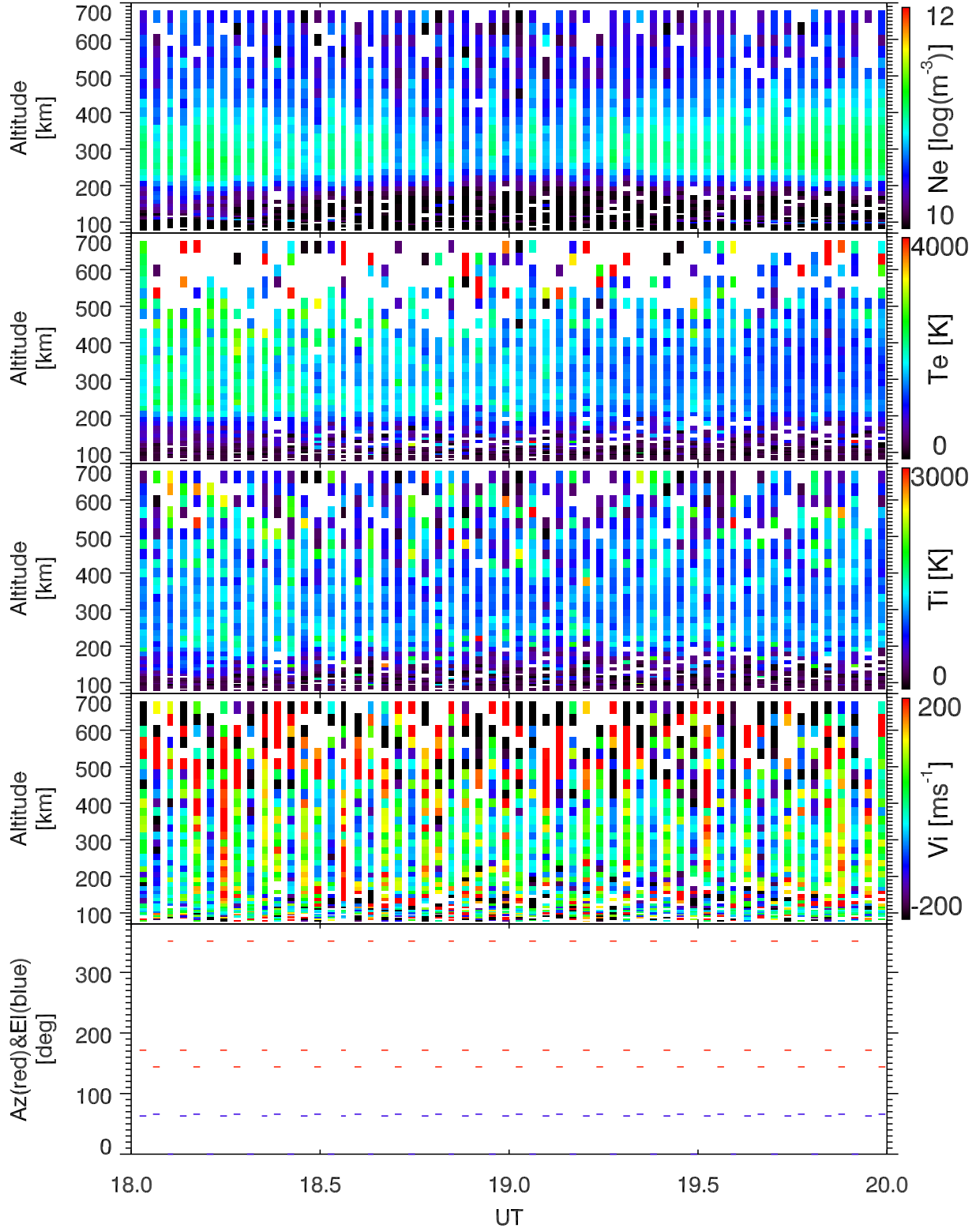
EISCAT 2005-09-23_18_20UT_steffe_ant@32m.
