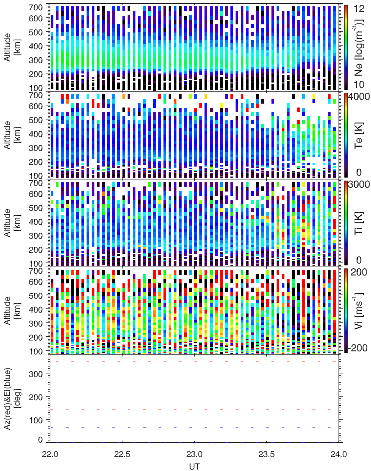
EISCAT 2005-09-24_22_24UT_steffe_ant@32m.
