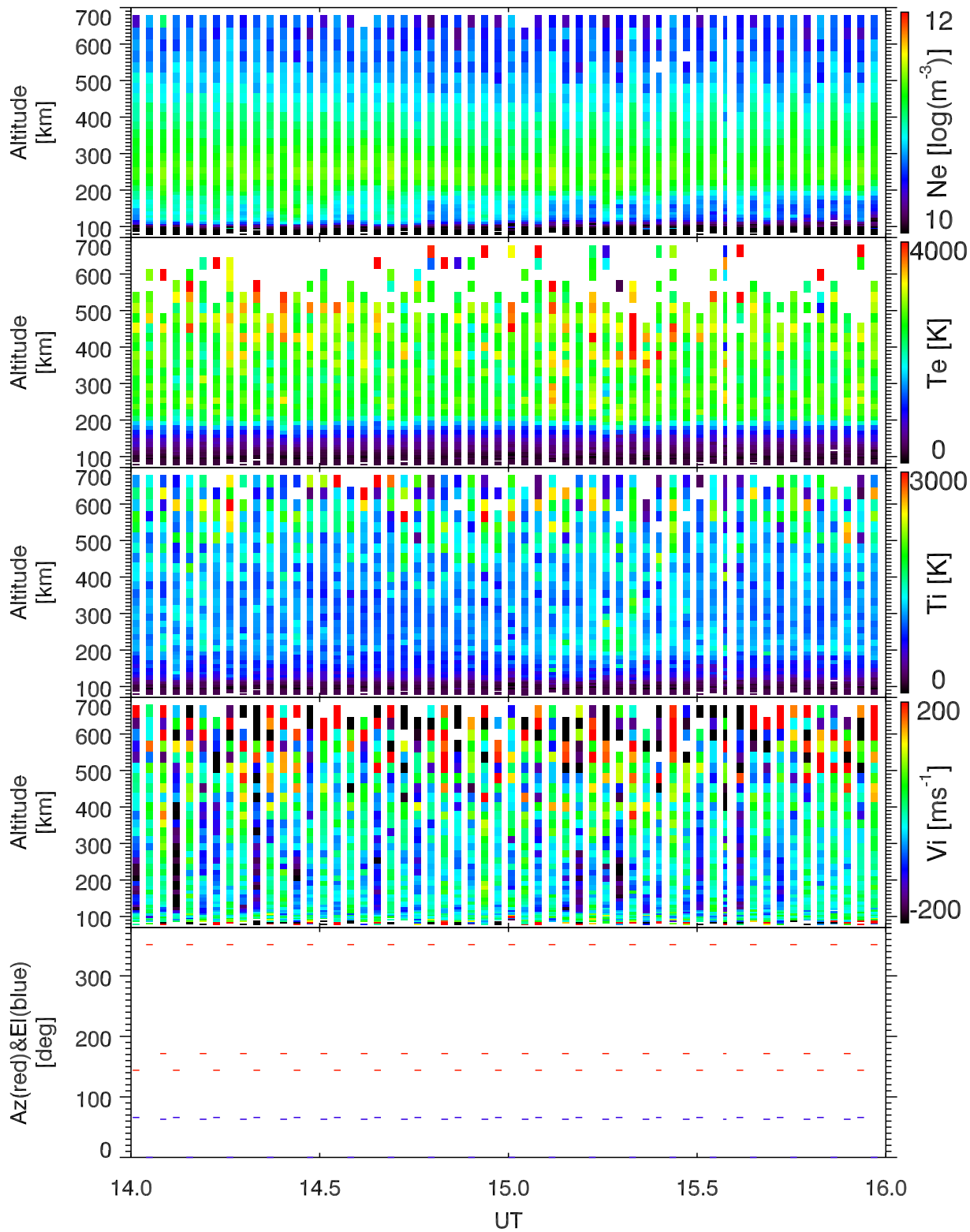
EISCAT 2005-09-25_14_16UT_steffe_ant@32m.
