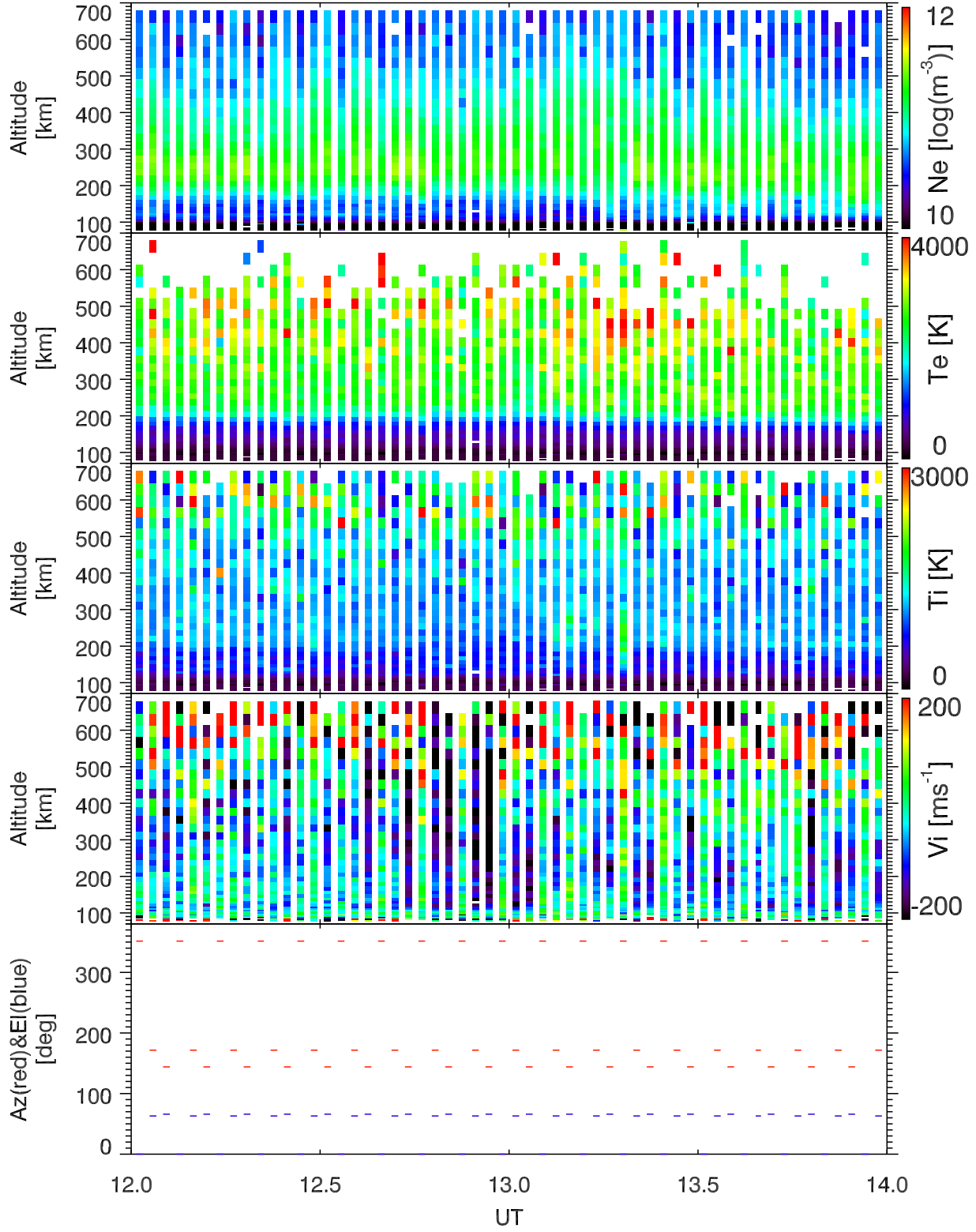
EISCAT 2005-09-26_12_14UT_steffe_ant@32m.
