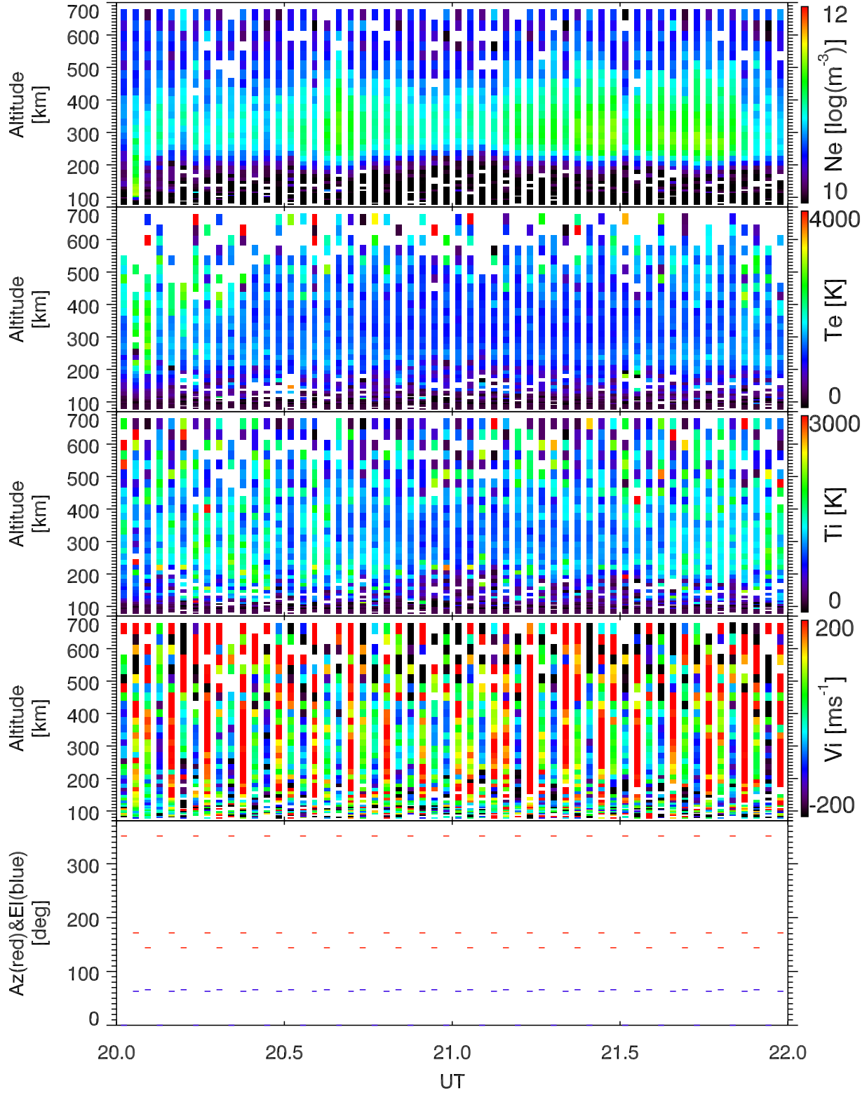
EISCAT 2005-09-26_20_22UT_steffe_ant@32m.
