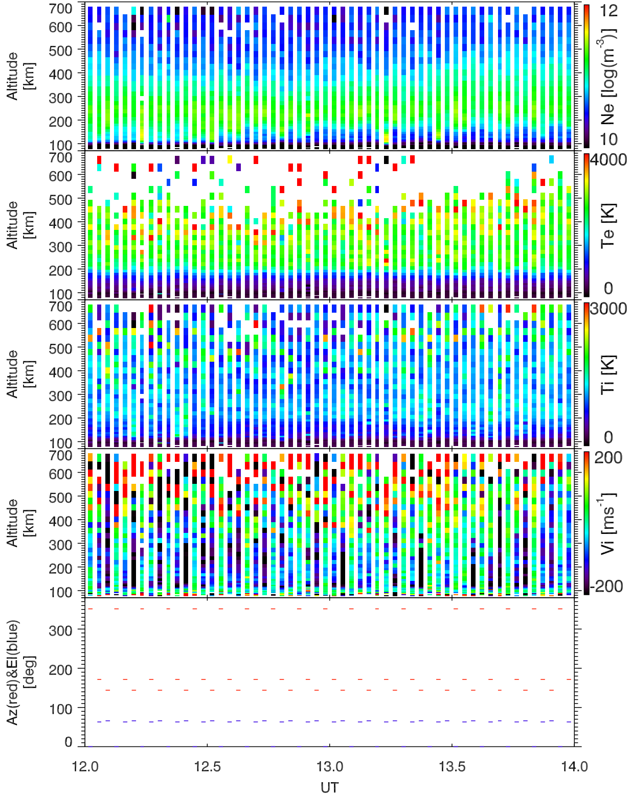
EISCAT 2005-09-27_12_14UT_steffe_ant@32m.
