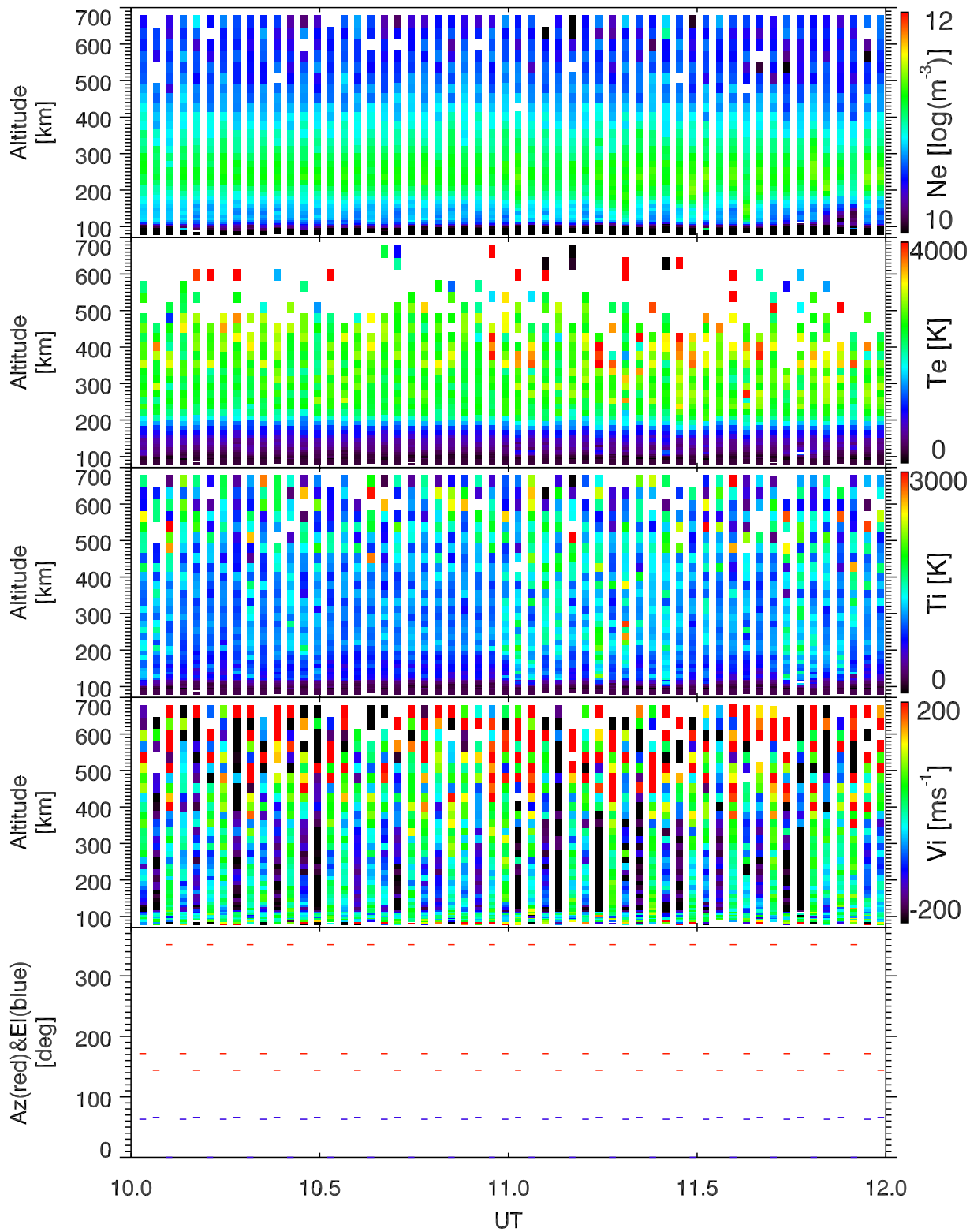
EISCAT 2005-09-28_10_12UT_steffe_ant@32m.
