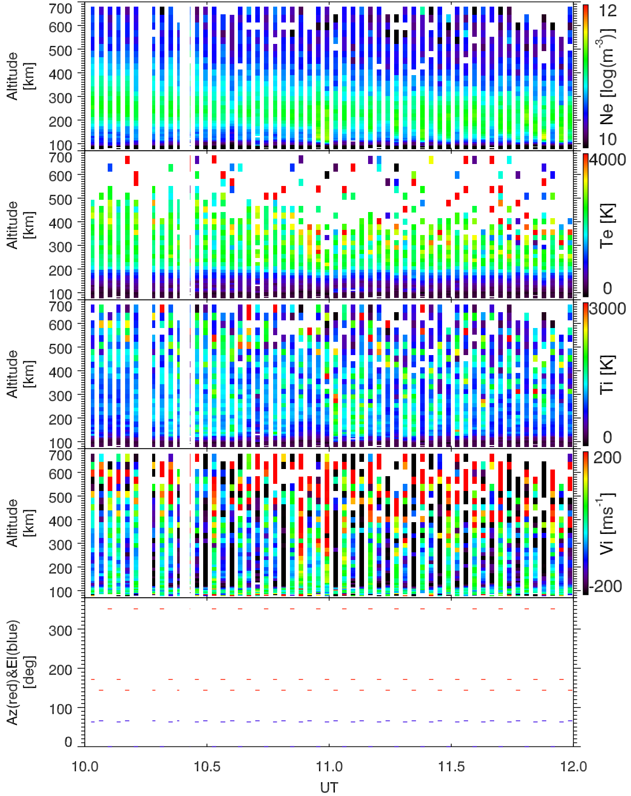
EISCAT 2005-09-29_10_12UT_steffe_ant@32m.
