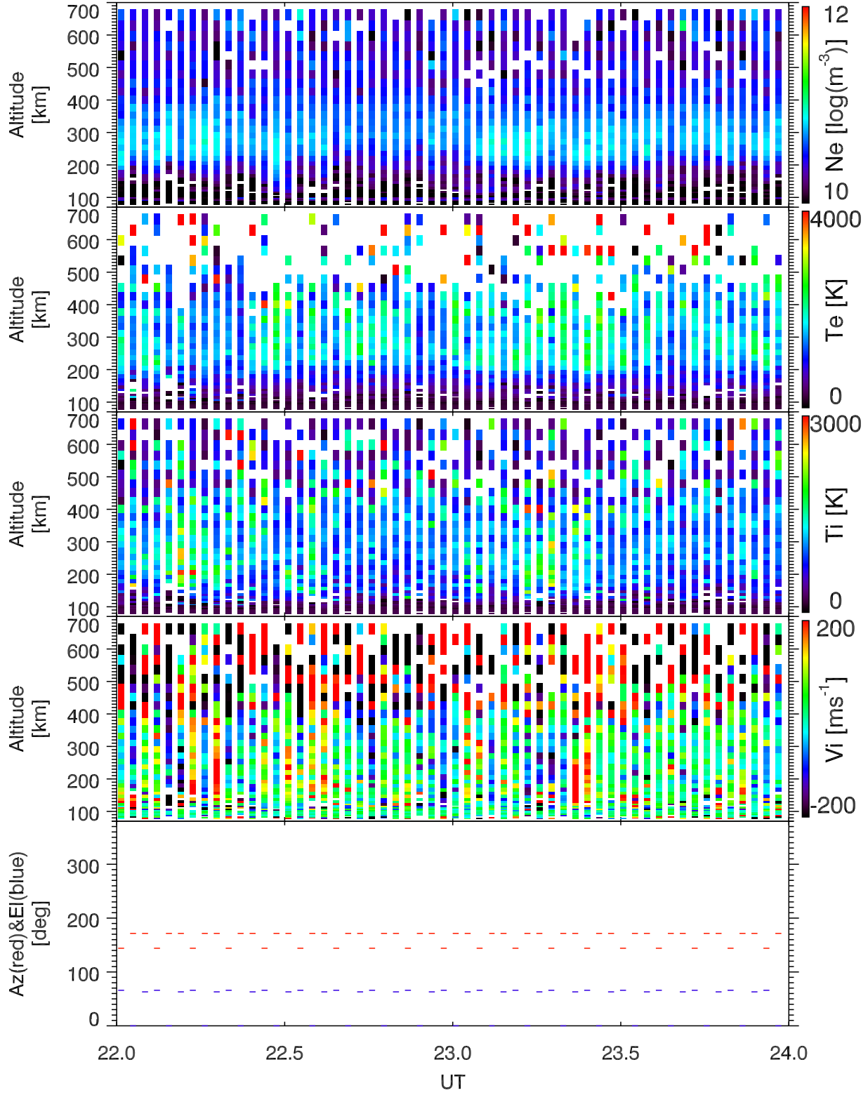
EISCAT 2005-09-29_22_24UT_steffe_ant@32m.
