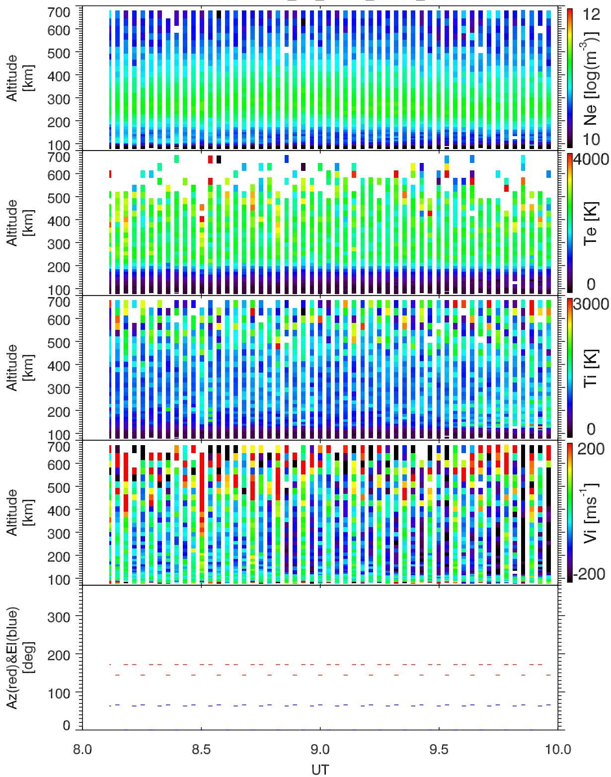
EISCAT 2005-09-30_08_10UT_steffe_ant@32m.
