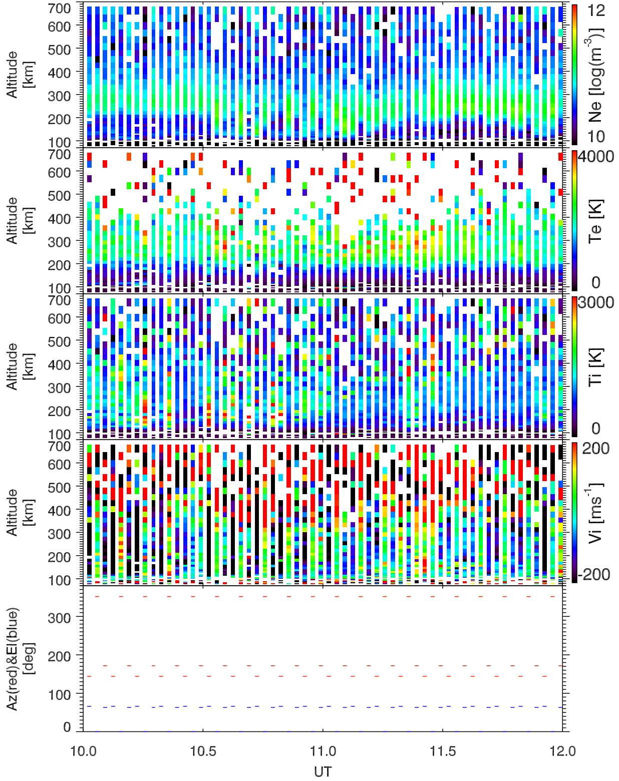
EISCAT 2007-02-07_10_12UT_steffe_ant@32m.
