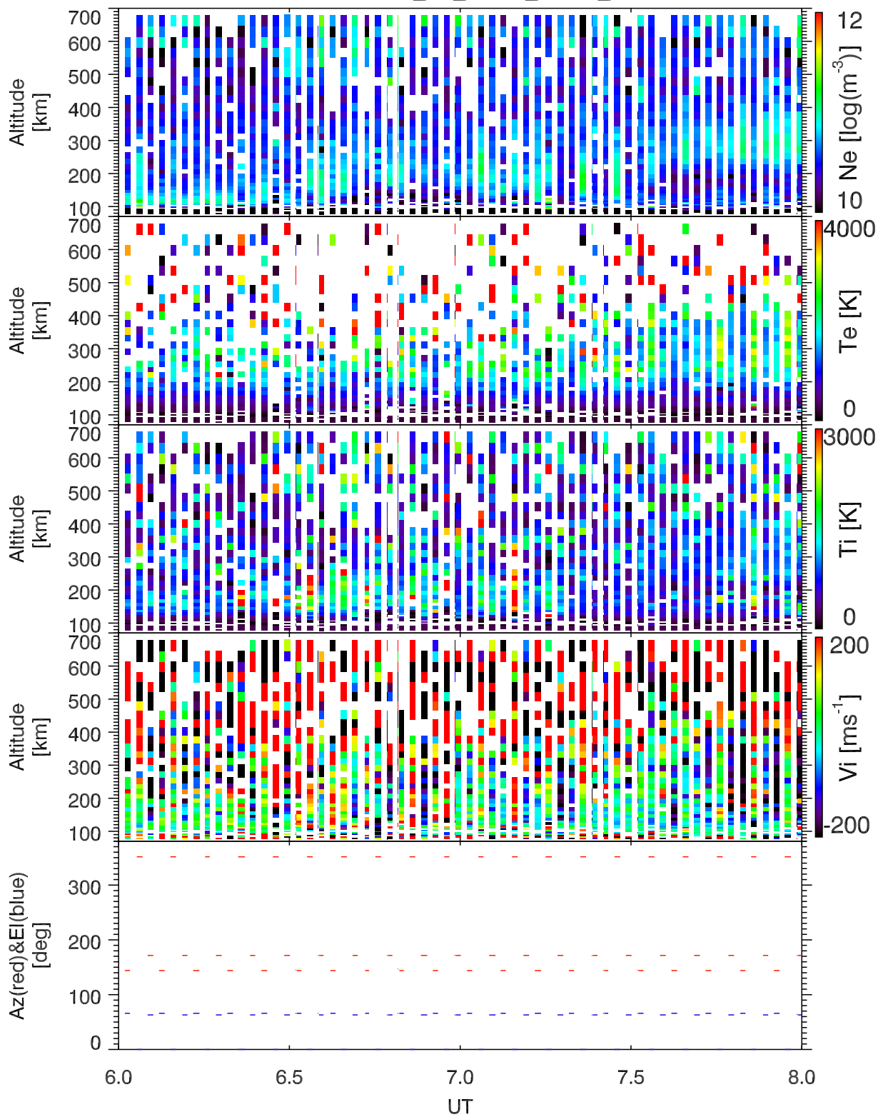
EISCAT 2007-02-08_06_08UT_steffe_ant@32m.
