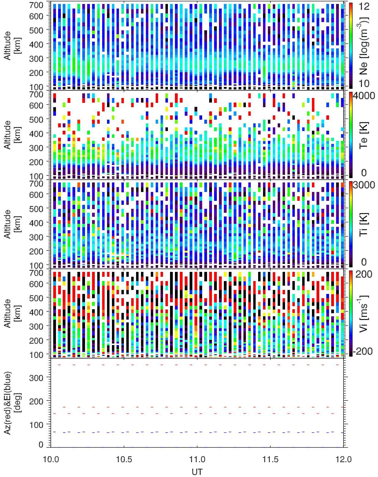
EISCAT 2007-02-08_10_12UT_steffe_ant@32m.
