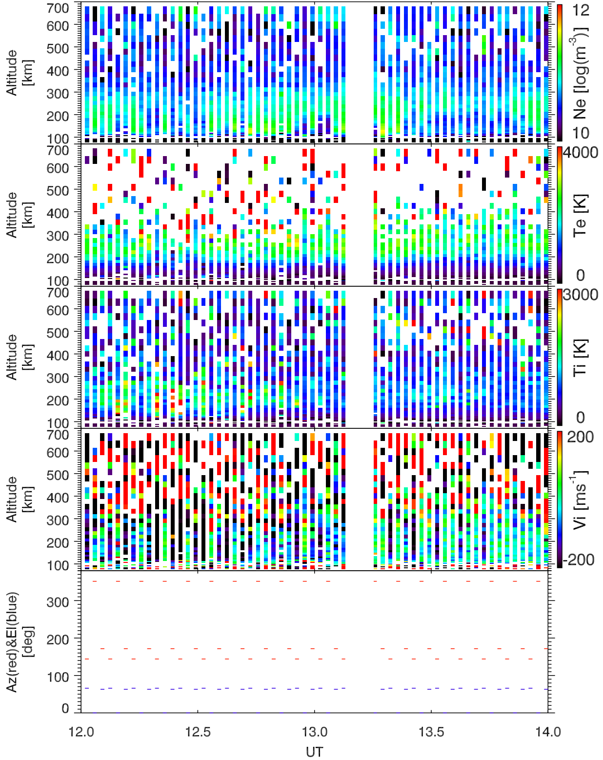
EISCAT 2007-02-08_12_14UT_steffe_ant@32m.
