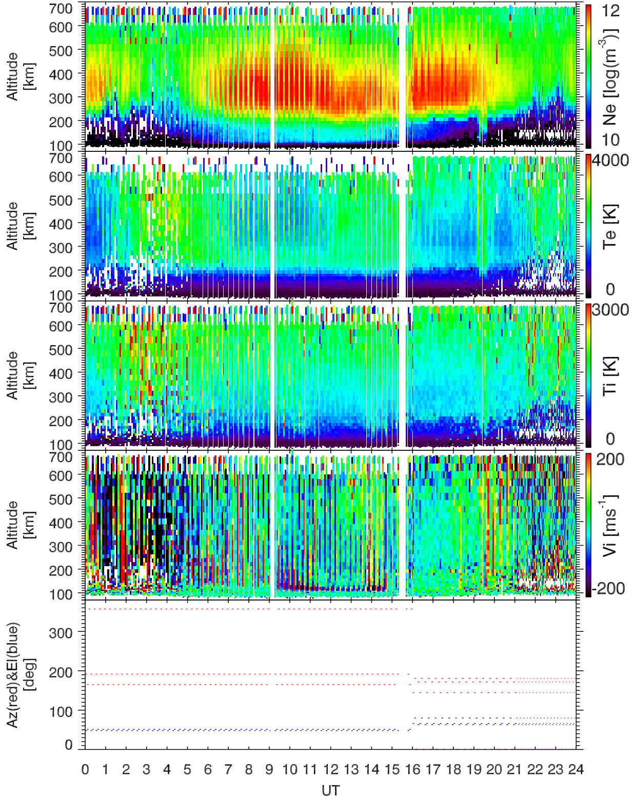
EISCAT 2000-03-17_00_24UT_gup3c_ant@32m.
