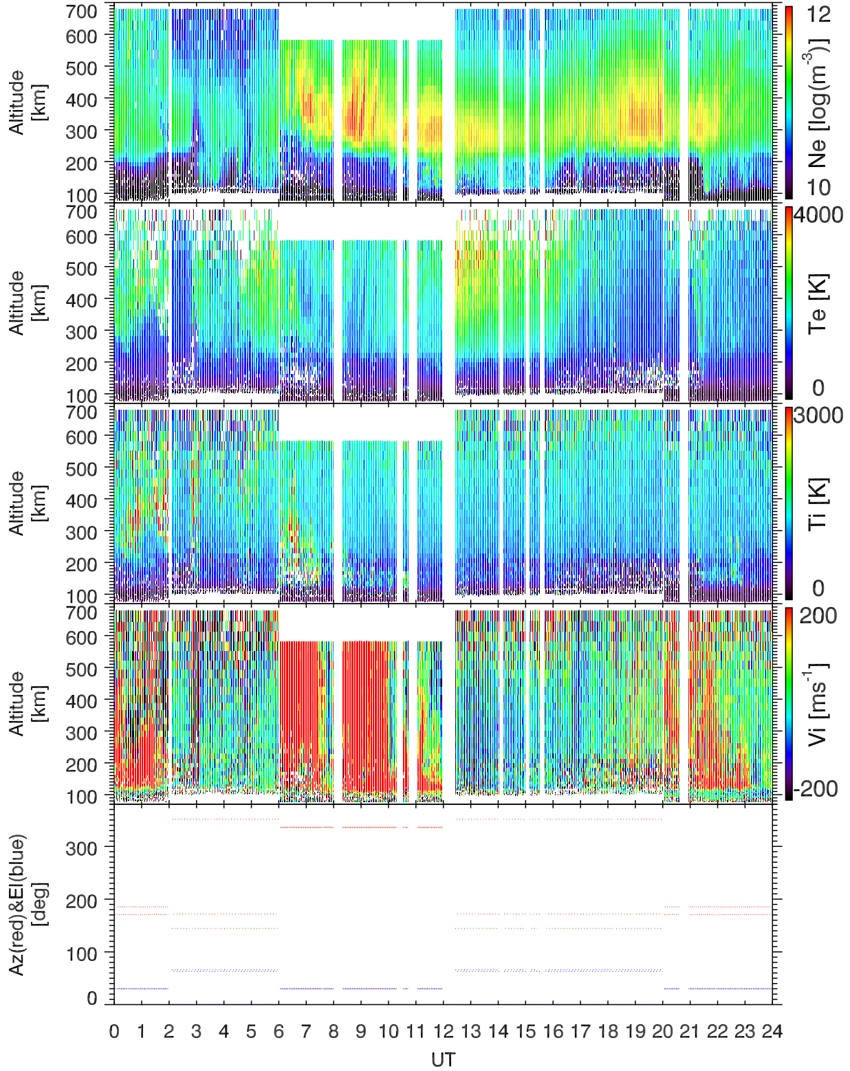
EISCAT 2001-02-21_00_24UT_tau0_ant@32m.
